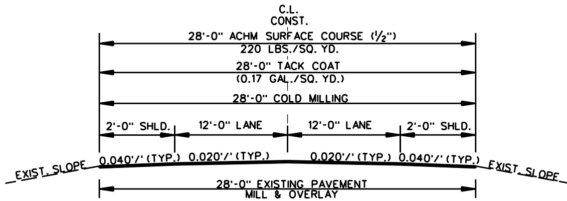
2 LANE OPEN SHOULDER MILL & OVERLAY STA. 100+00 TO STA. 104+22
