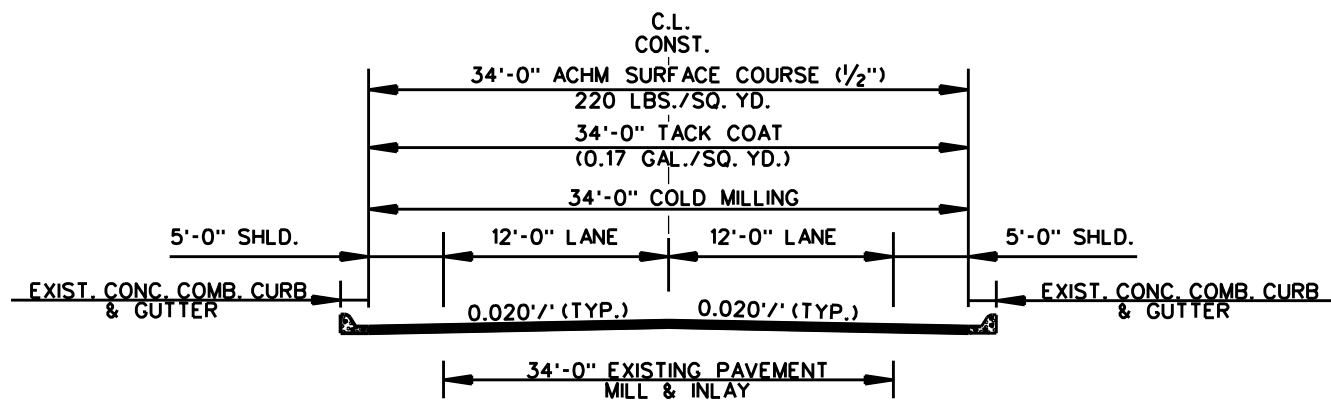
2 LANE CURB & GUTTER INLAY STA. 104+22 TO STA. 110+43 STA. 114+03 TO STA. 119+65
